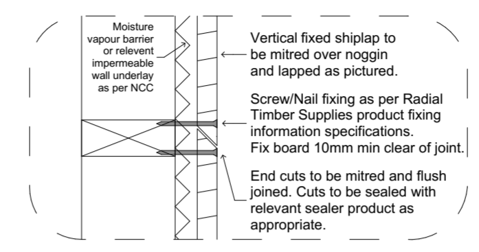
1.1 S02:A1 - Vertical Shiplap Mitre Join 1:5
